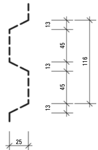
Detailprofilierung [mm]
