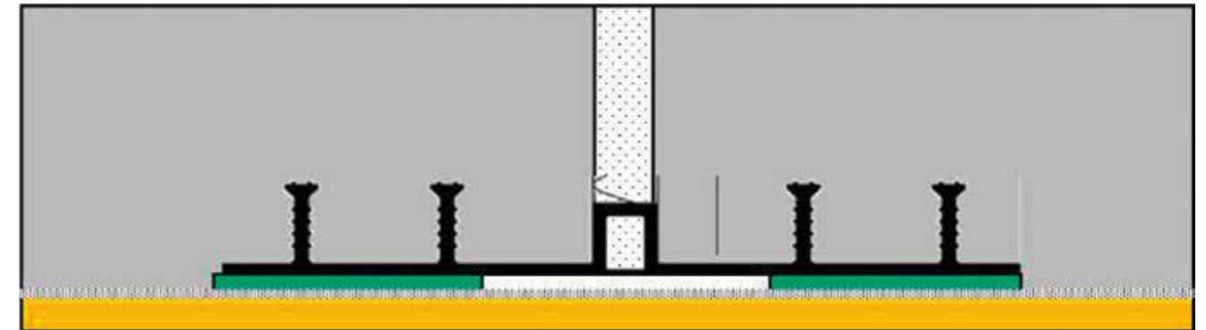
Sicherung einer Dehnfuge mit außenliegenden Fugenbändern, z. B. DFT Profile
